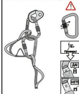
Рис. 4. Установка на карабин
